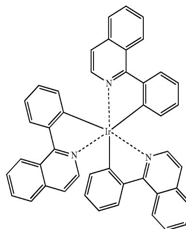
Ir(piq) 3
